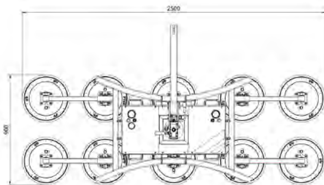
110kg - SWL 1000kg- Linientyp Lifter
