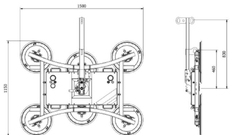
85kg - SWL 600kg- Spinnentyp Lifter
